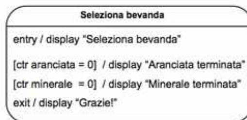
Figura 7. Uno stato con transizioni interne
