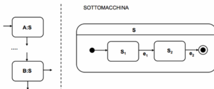
Figura 13. Una sottomacchina S richiamata da più punti di un diagramma a stati di più alto livello
